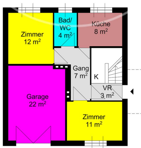
Skizze Erdgeschoss
