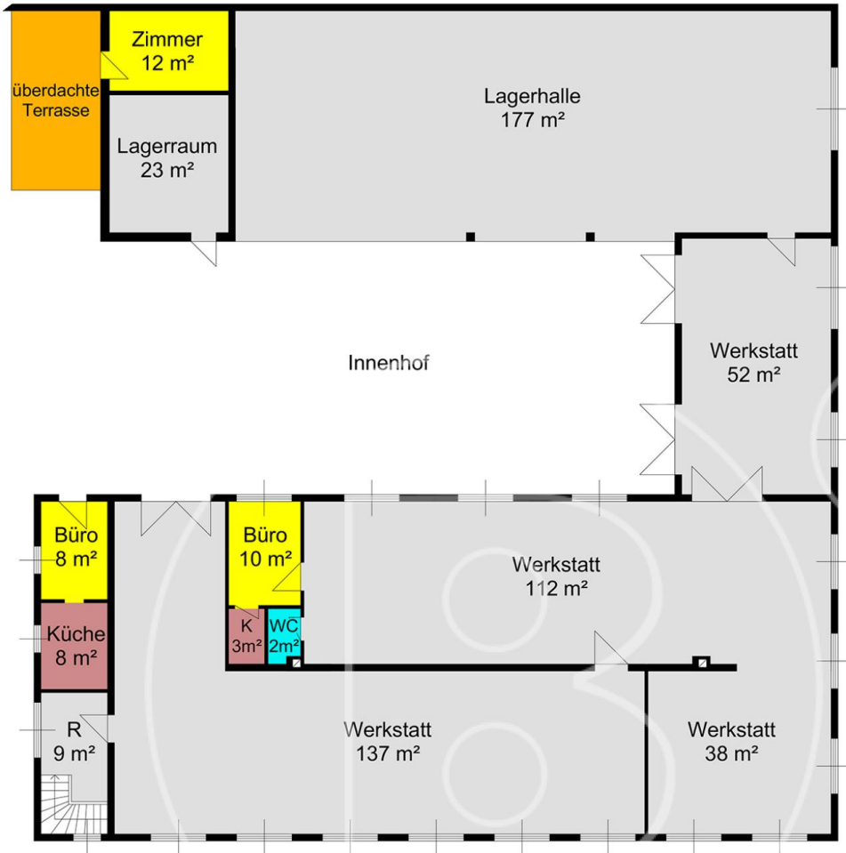
K ... Küche R ... Raum mit Abgang Keller Skizze Erdgeschoss
