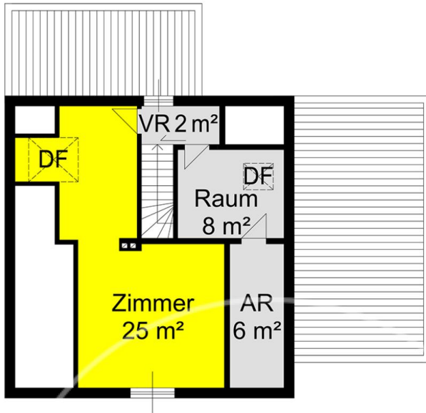
Skizze Dachgeschoss
