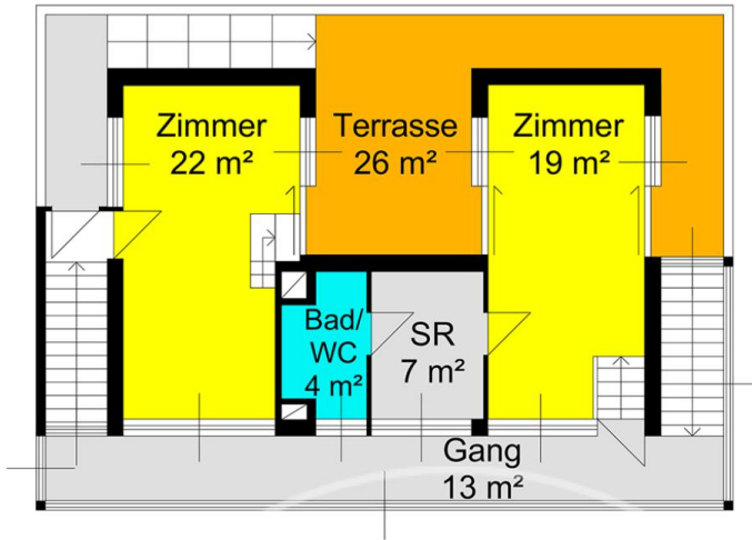
SR ... Schrankraum Skizze Obergeschoss
