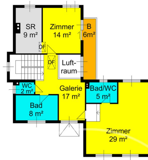
B ... Balkon DF ... Dachfenster SR ... Schrankraum Skizze Obergeschoss
