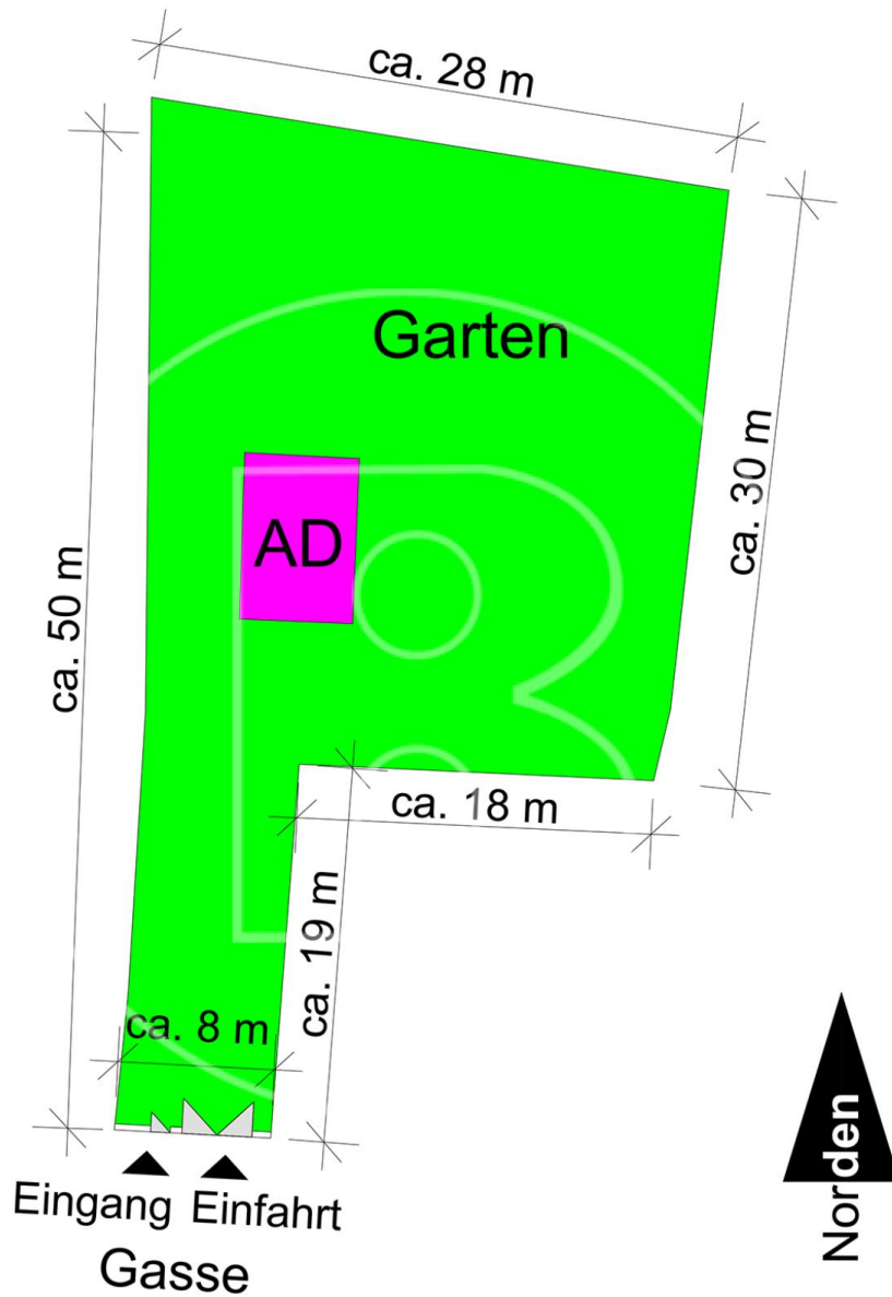
AD ... Altbestand Doppelgarage Skizze Lageplan
